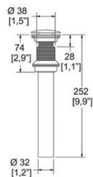
Dimensiones: vista lateral
